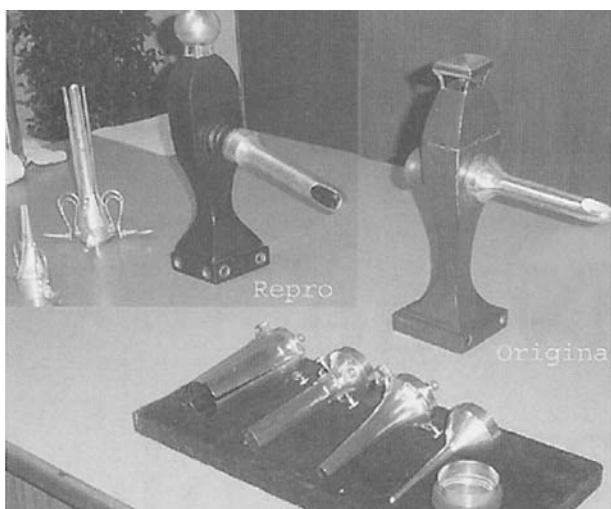
FIGURA 7. Conductor lumínico y espéculos.
