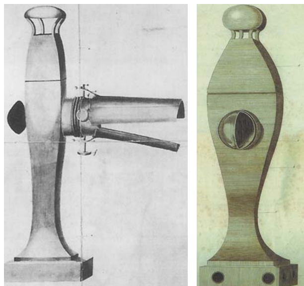
FIGURA 8 y 9. Conductor lumínico de perfil y de frente.
